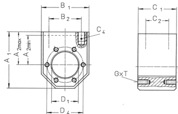
Bohrbild 3
