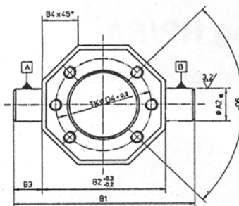
Bohrbild 1
