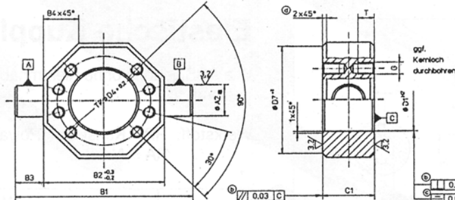
Bohrbild 2
